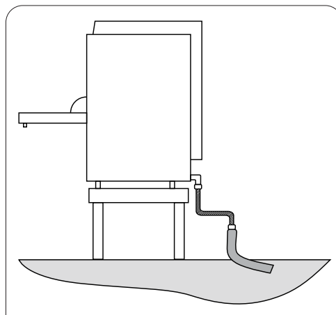
Drenaje por gravedad (Sólo para T316)
